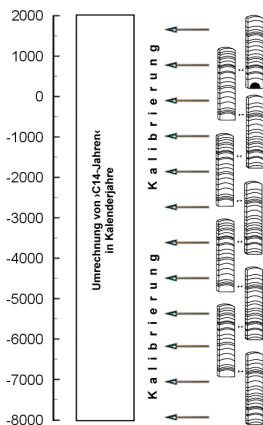
Bild 2: Mit dendrochronologischen Daten heraus aus dem Unwissen über die C14-Konzentration der Atmosphäre
